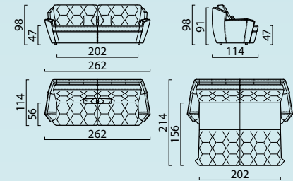
Диван Д140 «Кристалл» Side / Front / Top view
