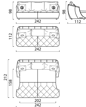
Диван-кровать ДКР 200 «Сальто 2» Front / Side / Top view
